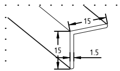
Cornière Aluminium 15x15
