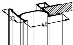
Profil Vertical : -Aluminium anodisé ou laqué
