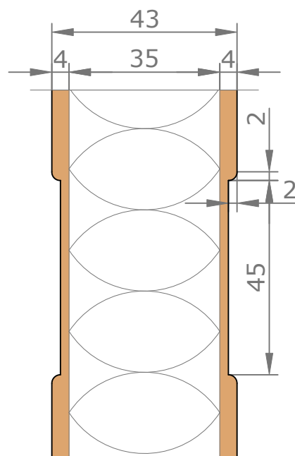
Détail de l'usinage
