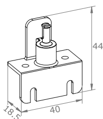
③b Support Amortisseur (Cezame)
