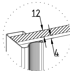
Vitre/Miroir : épaisseur 4 mm Panneau : épaisseur 12 mm
