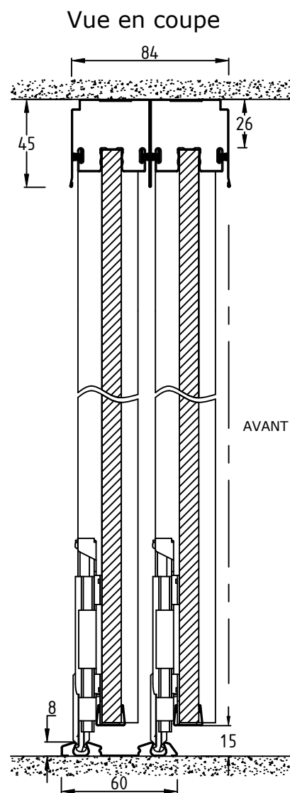
Vitre/Miroir : épaisseur 4 mm Panneau : épaisseur 12 mm
